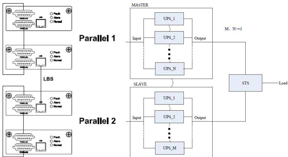
Рисунок 9 — Схема соединения изделий через LBS-кабель
