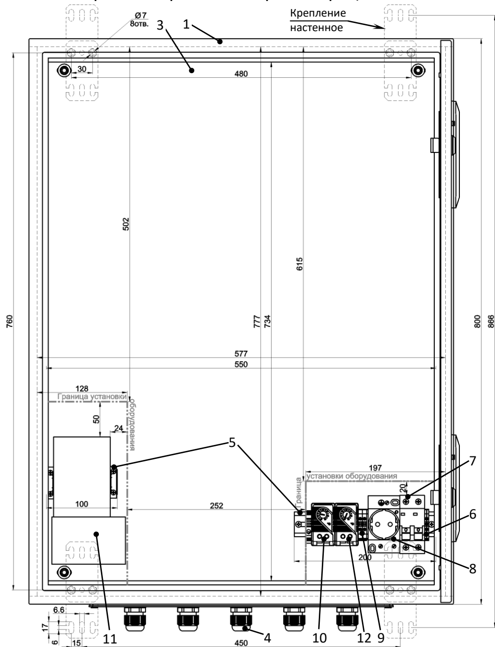
Рисунок 1 – Устройство шкафа
